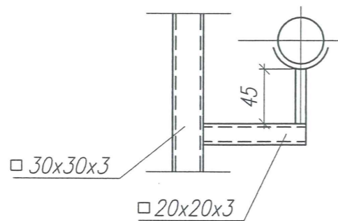
SPOSÓB PODPARCIA RUROCIĄGÓW
